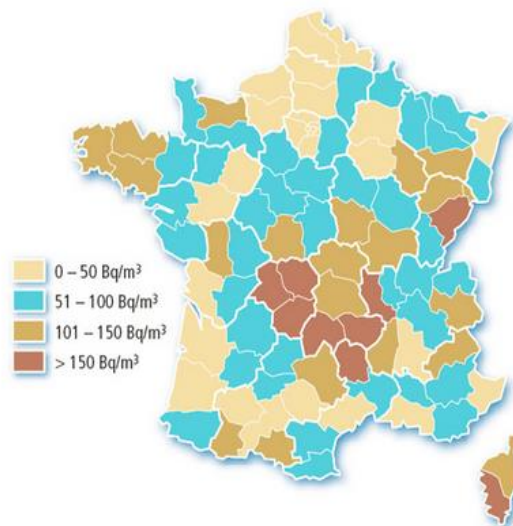
Moyenne par département des concentrations en radon dans l'air des habitations (en Bq/m³)
